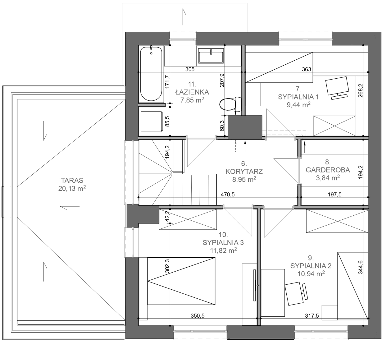
RZUT PIĘTRA
