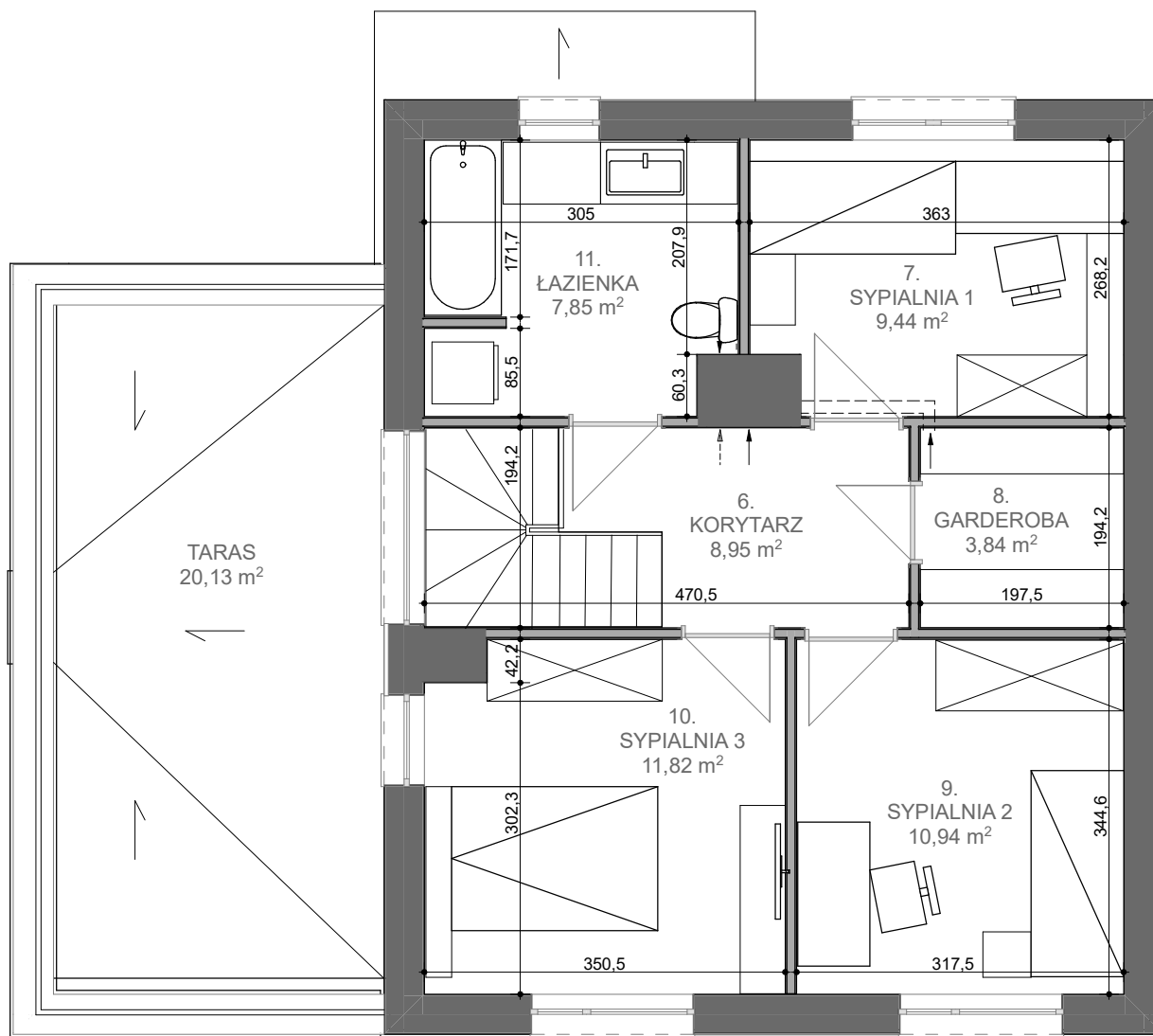
RZUT PIĘTRA
